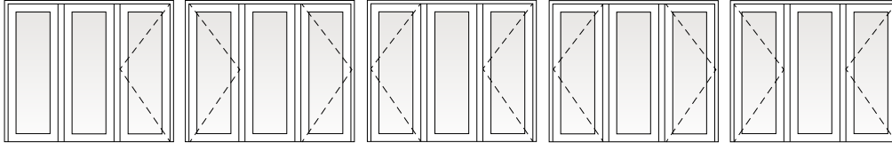
71168SSAL-3 71168ASARR-3 71168ASALL-3 71168ASALR-3 71168ASARL-3 711611SSAL-3 711611ASARR-3 711611ASALL-3 711611ASALR-3 711611ASARL-3 71180SSAL-3 71180ASARR-3 71180ASALL-3 71180ASALR-3 71180ASARL-3 711100SSAL-3 711100ASARR-3 711100ASALL-3 711100ASALR-3 711100ASARL-3
