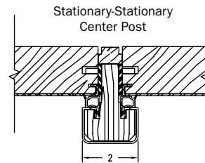
Astragal
