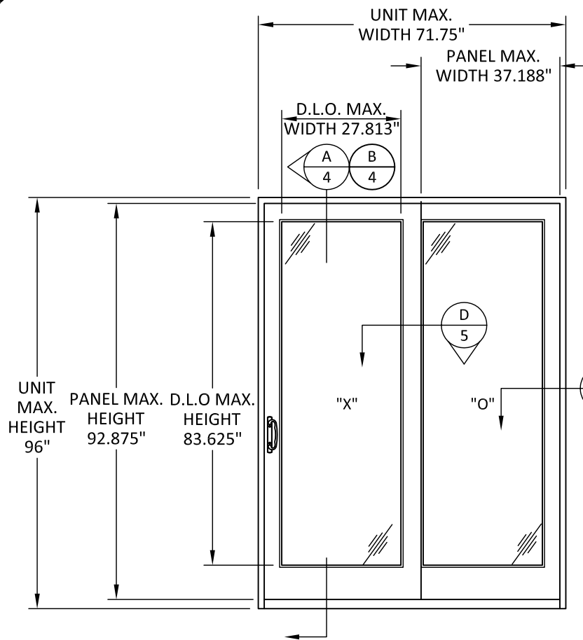
ELEVATION
