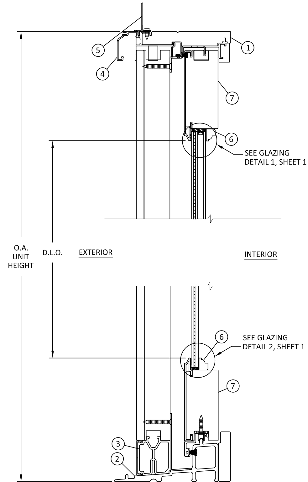
A 4 VERTICAL SECTION FIN
