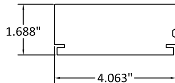
10 JAMB CAP FLASHING ALUMINUM
