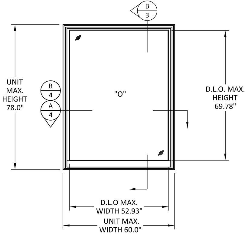
ELEVATION
