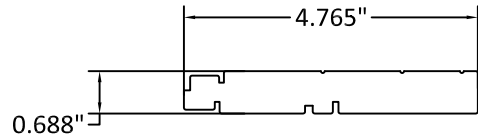
10 HEAD JAMB
