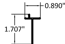
70 NAIL FIN
