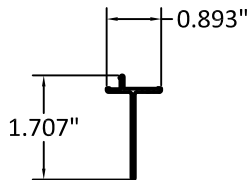
70 NAIL FIN
