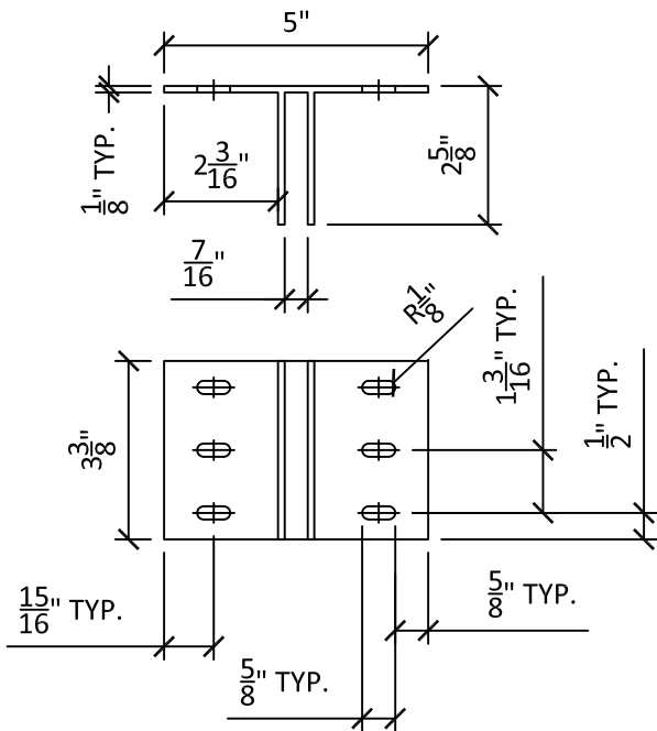
MULLION CLIP - F1 ALUMINUM (6063-T6)
