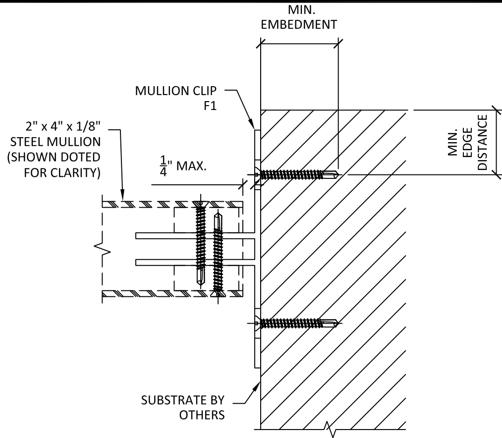
A 3 VERTICAL SECTION CLIP F1 INSTALLATION
