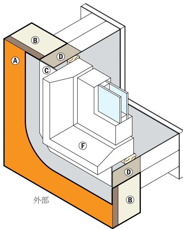
使用結構緊固支撐件安裝的窗或門
