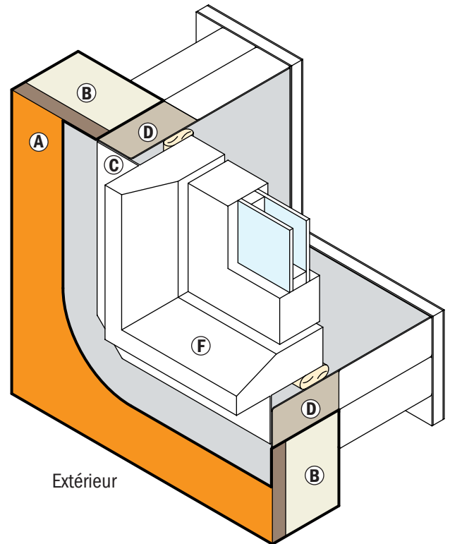
Fenêtre ou porte installée avec pièces de support fixées structuellement
