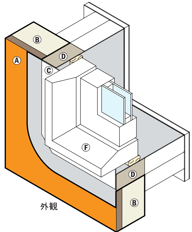
構造的に固定されたサポートピースで取り付けられた窓またはドア
