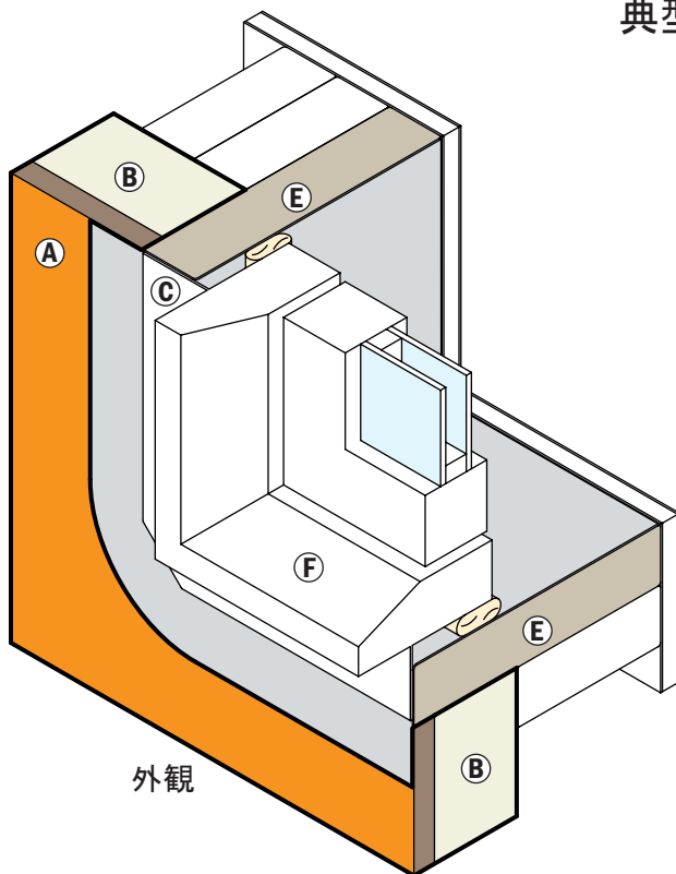
貫通構造サポートで取り付けられた窓またはドア
